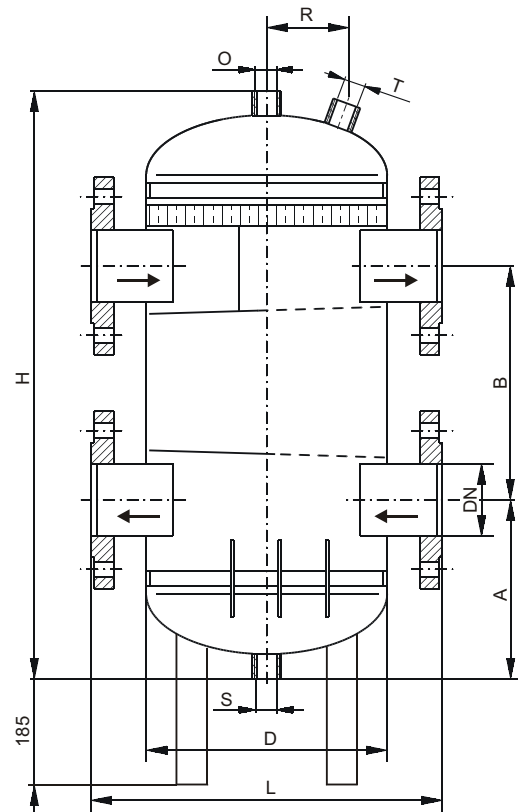
Sprzęgło hydrauliczne typ SPP (wymiar)
