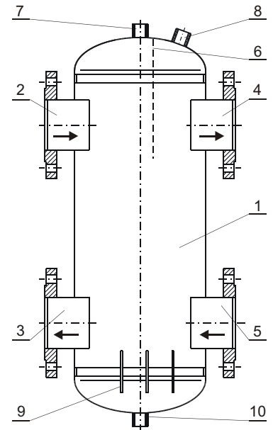
Sprzęgło hydrauliczne typ SP (budowa)
